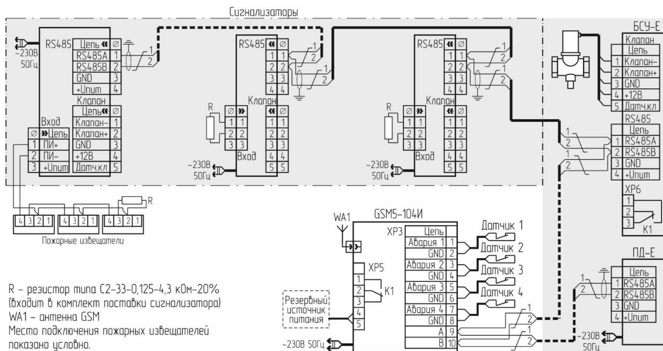
Рисунок IV.2 – Система с RS485 и групповой защитой. Типовая схема соединений.
