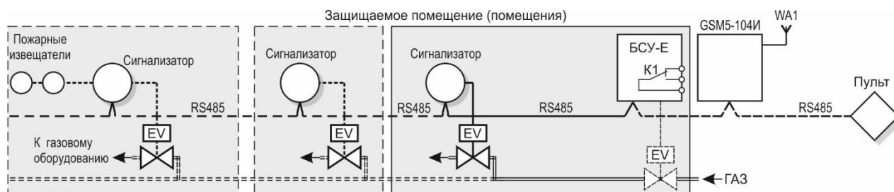
Рисунок IV.3 - Структура системы с RS485 и индивидуальной защитой.
