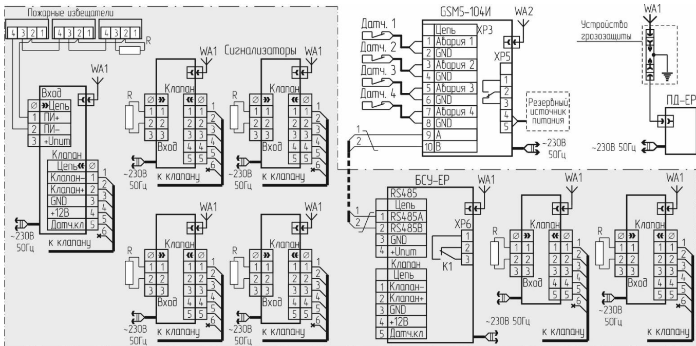
Рисунок IV.11 - Структура системы с радиоканалом (звезда) и индивидуальной защитой.
