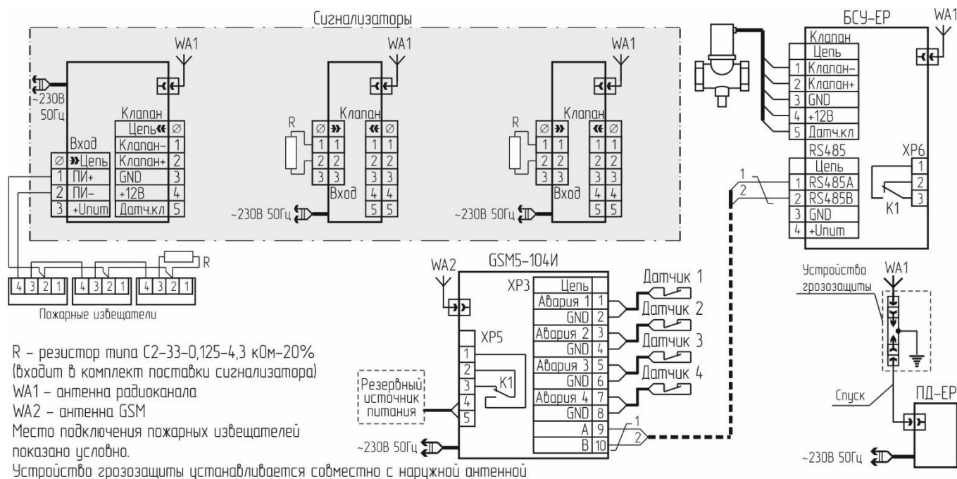
Рисунок IV.6 – Типовая схема соединений системы с радиоканалом (линия) и групповой защитой.
