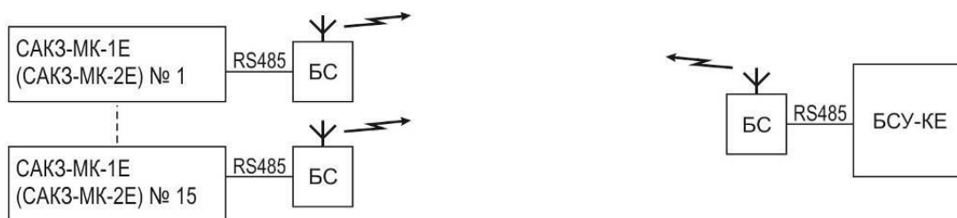
а) блок-схема
