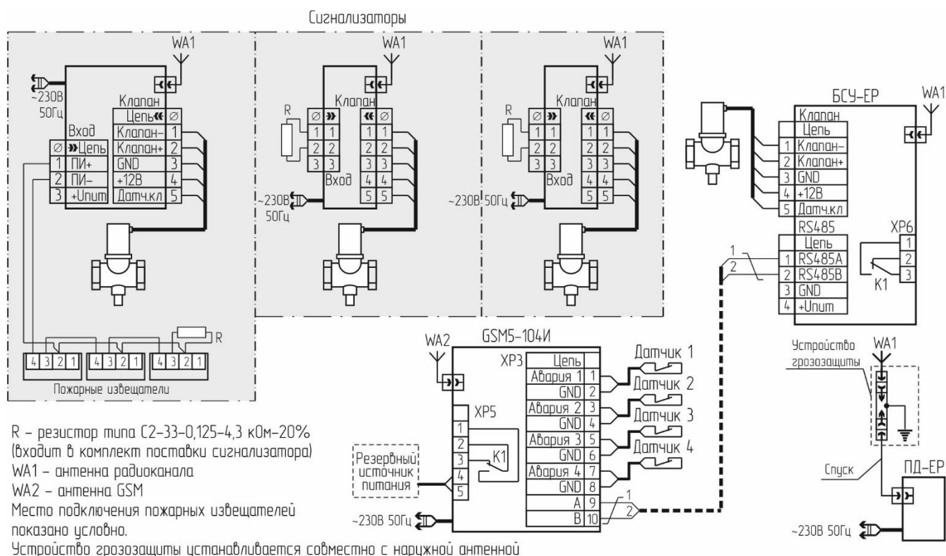
Рисунок IV.8 – Типовая схема соединений системы с радиоканалом (линия) и индивидуальной защитой.
