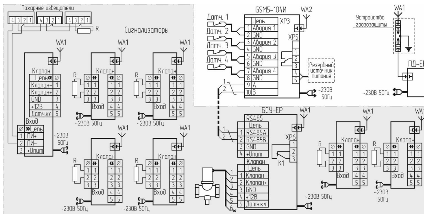
Рисунок IV.9 - Структура системы с радиоканалом (звезда) и групповой защитой.
