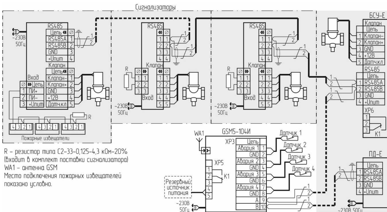
Рисунок IV.4 – Типовая схема соединений системы с RS485 и индивидуальной защитой.
