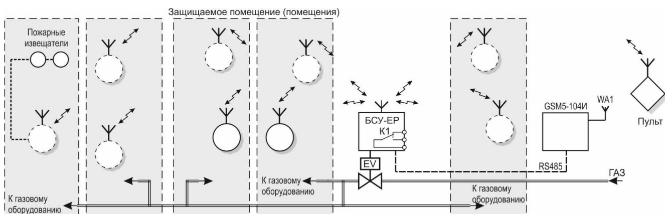
Рисунок IV.9 - Структура системы с радиоканалом (звезда) и групповой защитой.
