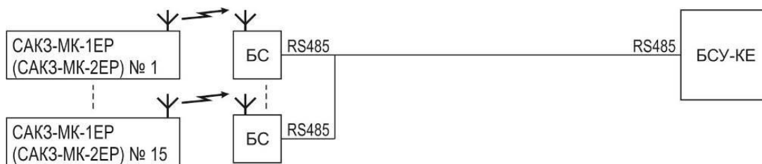
а) блок-схема
