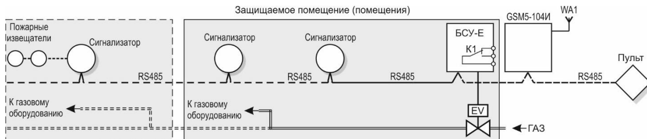
Рисунок IV.1 – Структура системы с RS485 и групповой защитой
