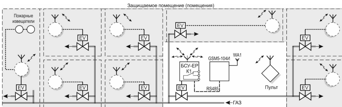
Рисунок IV.11 - Структура системы с радиоканалом (звезда) и индивидуальной защитой.
