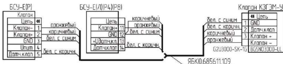
Рисунок Б.1 – Схема подключения клапана КЗГЭМ-У с разъемом BG5NO3000-UL.
