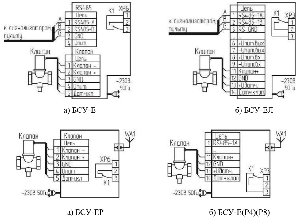
Рисунок 2 – Типовые схемы включения
