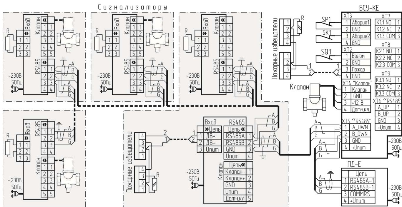
Рисунок 12 – Структура системы с интерфейсом RS485.
