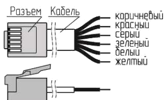
Вилка на кабель TP6P6C (цвета проводов)
