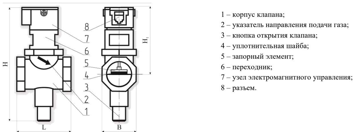
Рисунок 3 – Внешний вид клапана КЗЭУГ.
