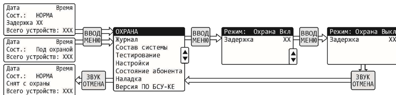
Рисунок 8 – Порядок действий для отключения режима охраны.
