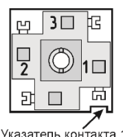
Розетка G2U3000-SK-1G
