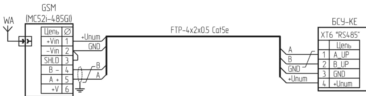
Рисунок Г.2 – Схема подключения GSM-извещателя MC52i-485GL.
