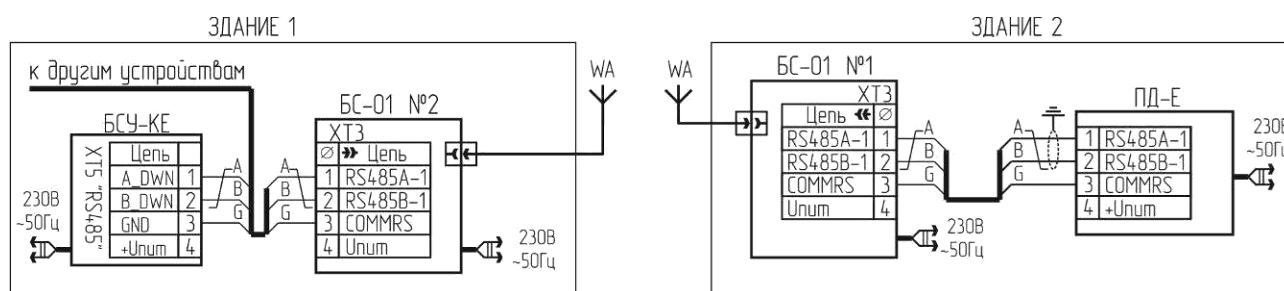
Рисунок 19 – Схема подключения удаленного пульта ПД-Е
