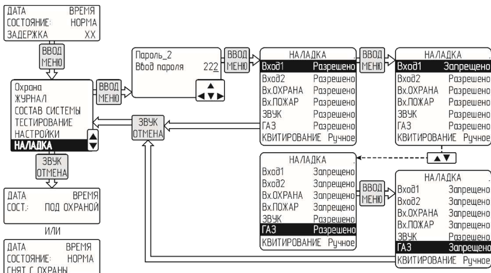
Рисунок 12 – Меню «Наладка»
