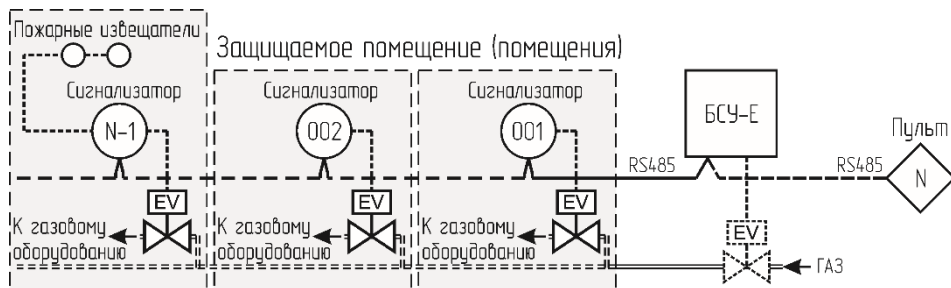
Рисунок 9 – Структура системы с RS485 и индивидуальной защитой.
