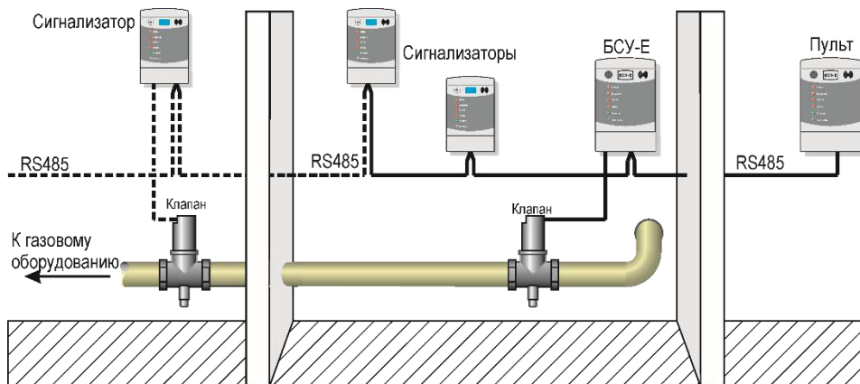
Рисунок А.1 – Пример схемы размещения системы с интерфейсом RS485.
