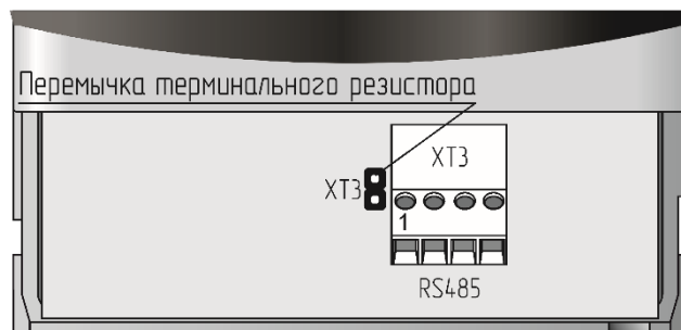
Рисунок Б.3 – Расположение разъемов в клеммном отсеке.
