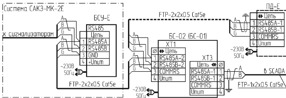
Рисунок Г.1 – Подключение системы САКЗ-МК-2Е к SCADA
