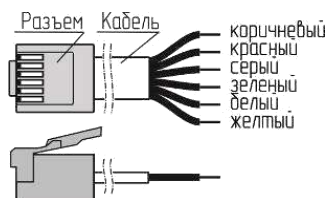
Вилка на кабель TP6P6C (цвета проводов)
