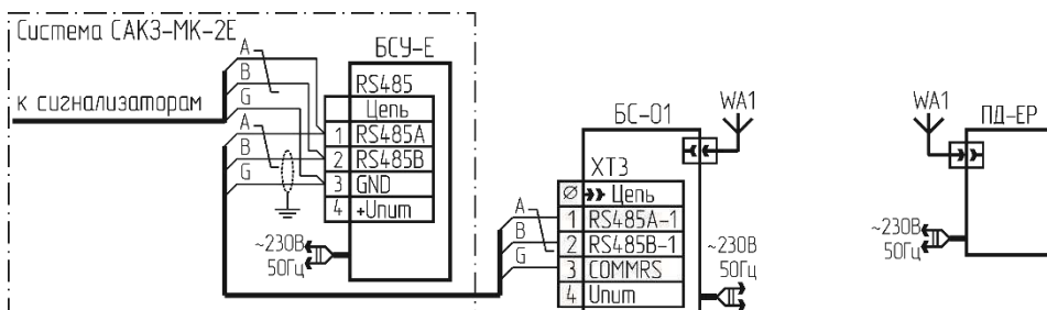
Рисунок В.5 – Схема подключения сигнализаторов исполнения «24» и пульта ПД-ЕВ к источнику вторичного электропитания.
