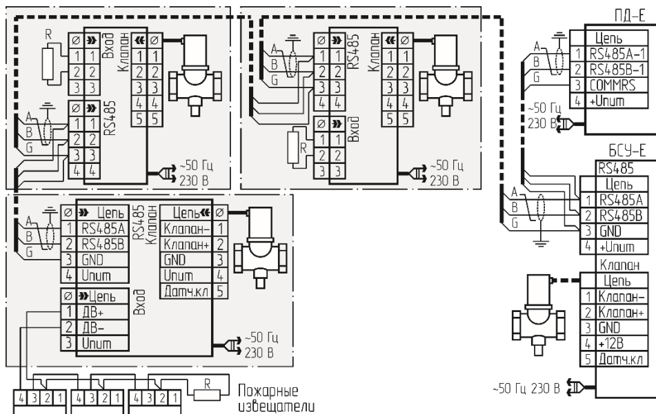
Рисунок 9 – Структура системы с RS485 и индивидуальной защитой.
