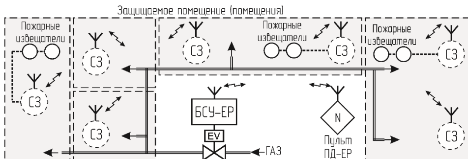
Рисунок 11 – Структура системы с радиоканалом и групповой защитой.
