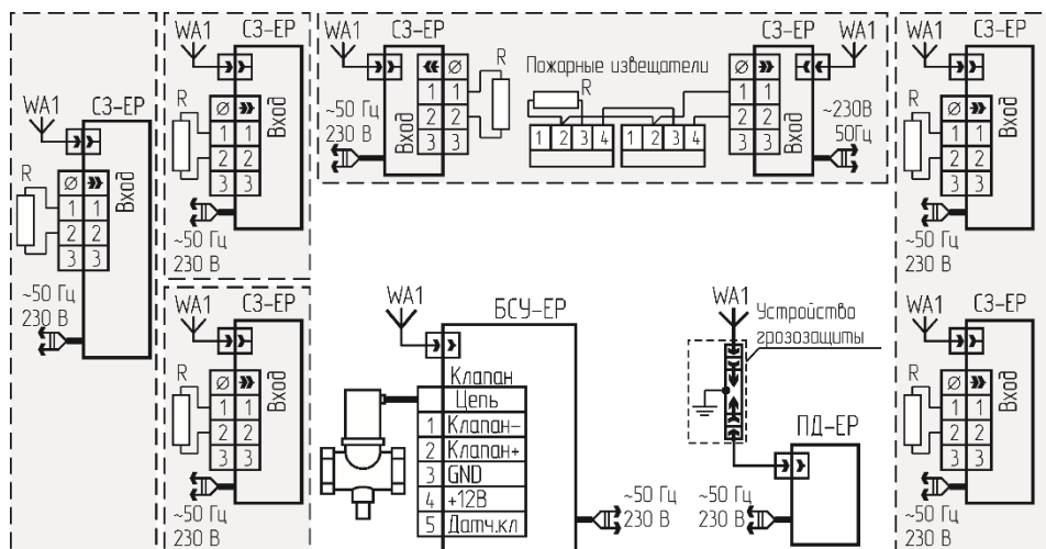
Рисунок 11 – Структура системы с радиоканалом и групповой защитой.
