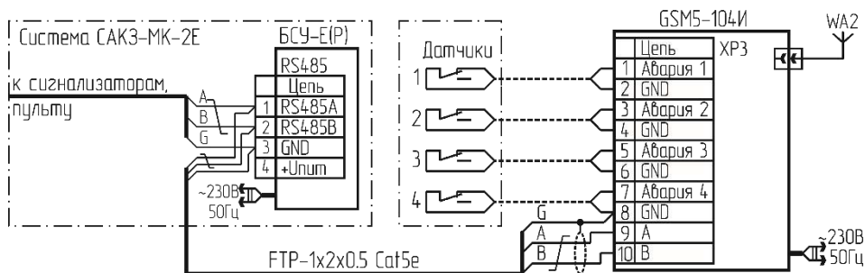
Рисунок В.7 – Схема подключения извещателя GSM5-104И
