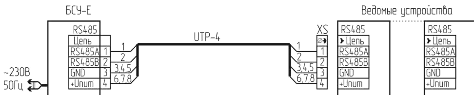
Рисунок 6 – Схема соединений для программирования адресов
