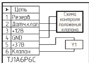
3 – Клапан КЗЭУГ.
