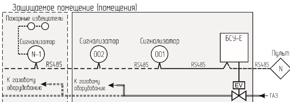
Рисунок 7 – Структура системы с RS485 и групповой защитой.
