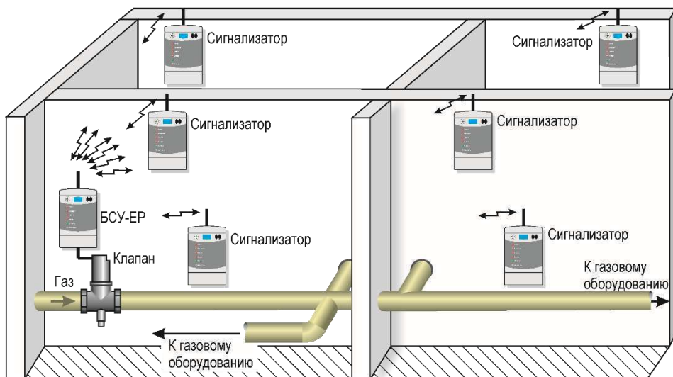
Рисунок А.2 – Пример схемы размещения системы с радиоканалом.
