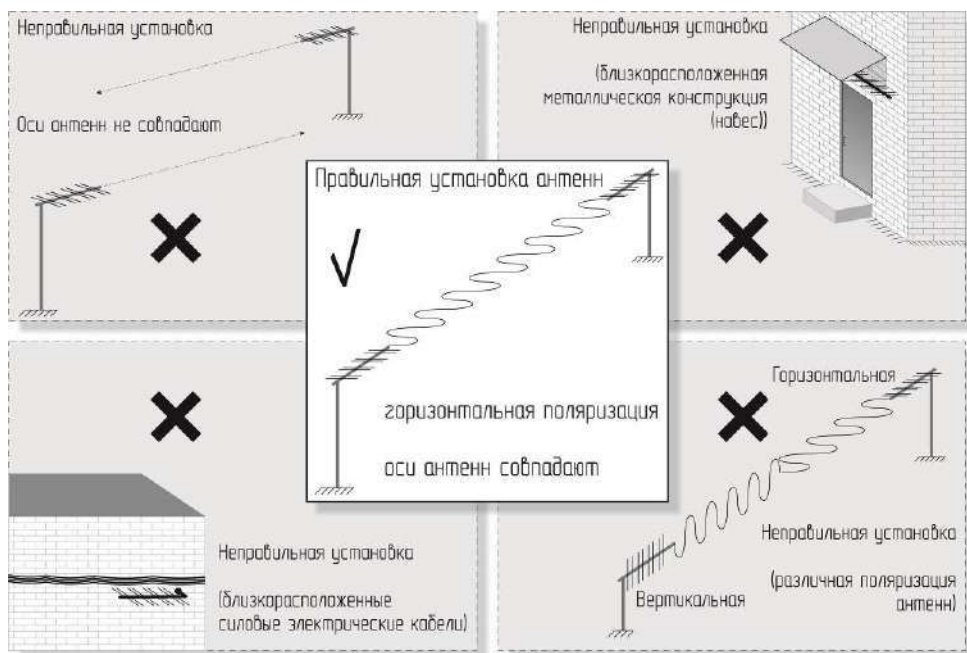
Рисунок Б.2 – Установка направленных антенн
