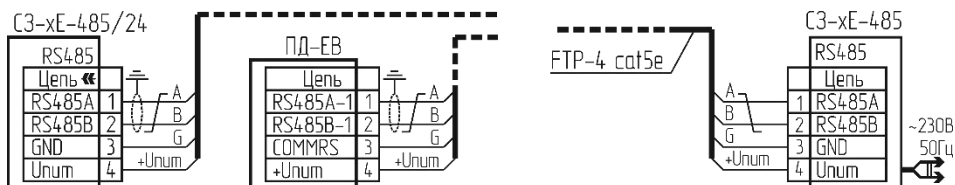
Рисунок В.3 – Нумерация контактов разъемов. Вид со стороны пайки (монтажа).
