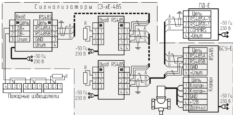
Рисунок 8 – Схема соединений системы с RS485 и групповой защитой.
