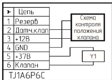
Рисунок 3 – Клапан КЗЭУГ.
