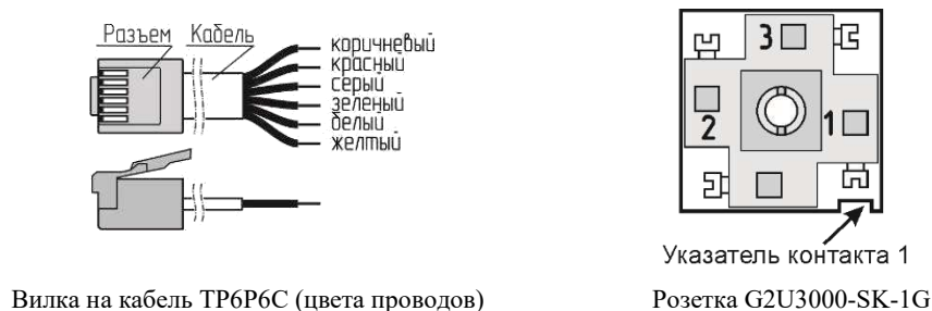
Рисунок В.3 – Нумерация контактов разъемов. Вид со стороны пайки (монтаж).
