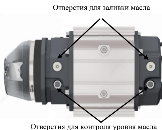
Рисунок 16. Заливка и контроль уровня масла при установке счетчика G10-G400 на вертикальном участке трубопровода
