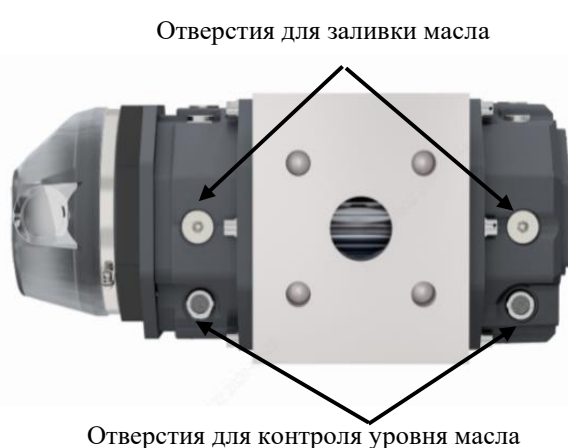
Рисунок 15. Заливка и контроль уровня масла при установке счетчика G10-G400 на горизонтальном участке трубопровода
