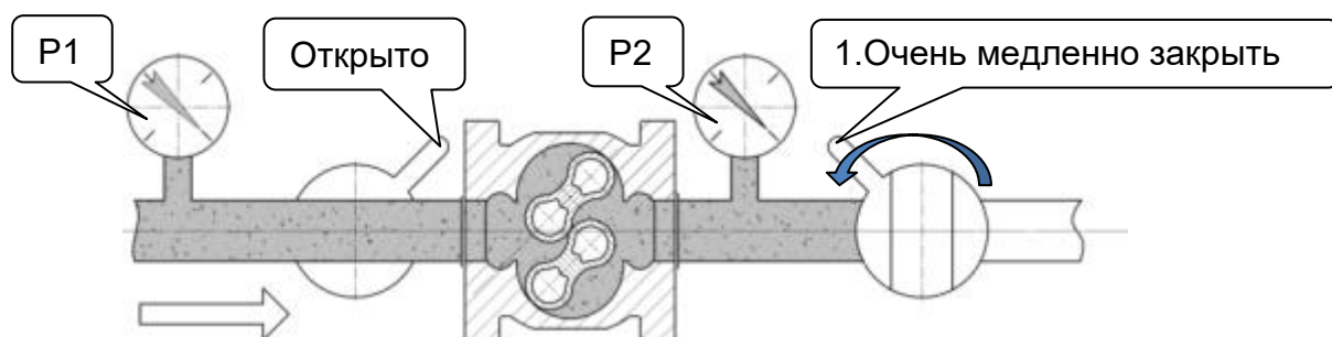
Рисунок 11. Начало остановки счетчика
