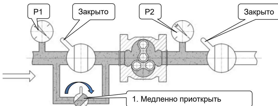
Рисунок 8. Открытие крана перепускного канала
